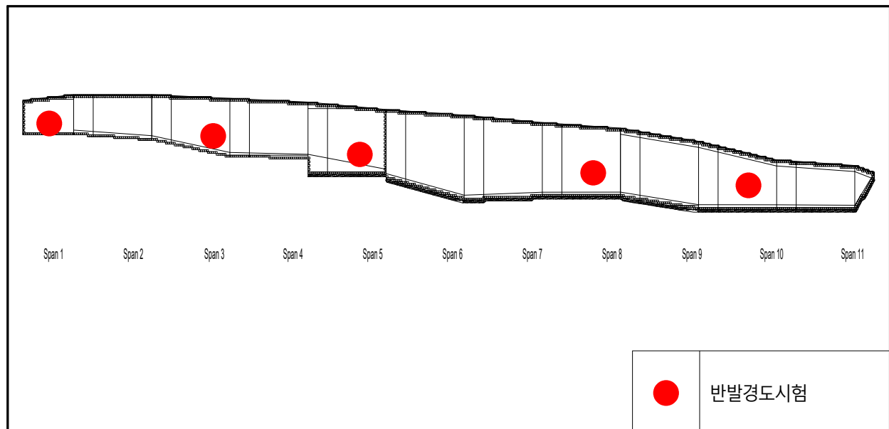
【그림 69.6】 콘크리트 재료시험 조사 위치도
