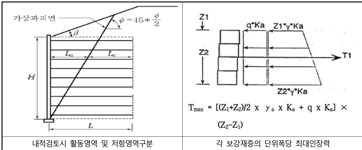
【그림 69.11】 토압작용 모식도
