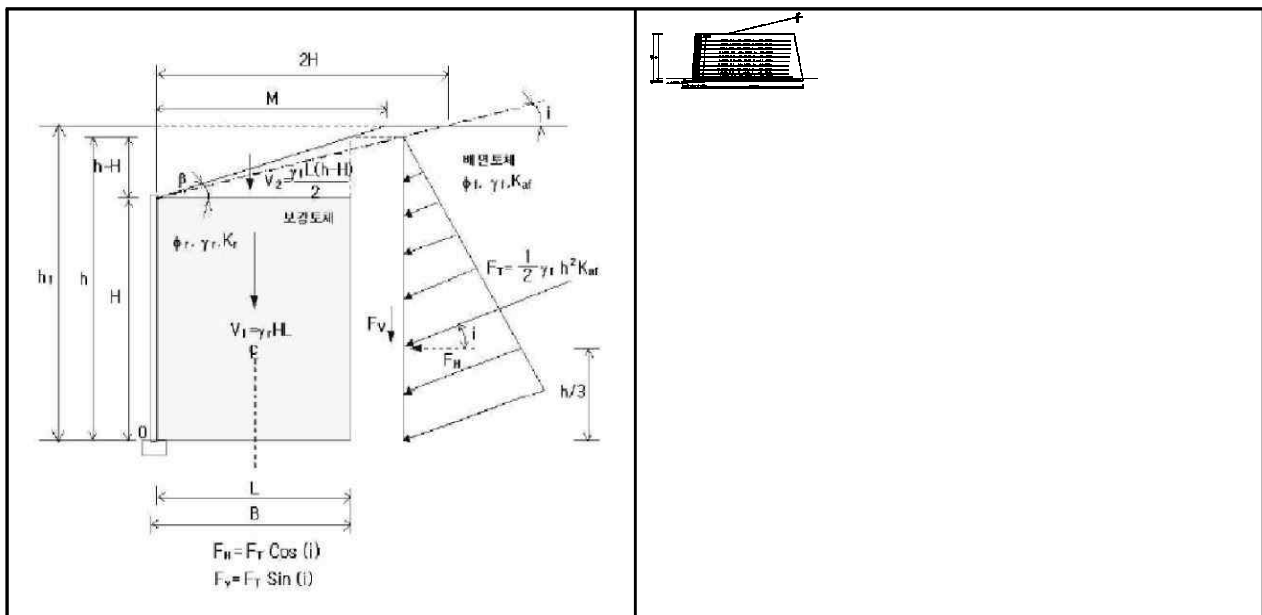
【그림 69.10】 검토단면도
