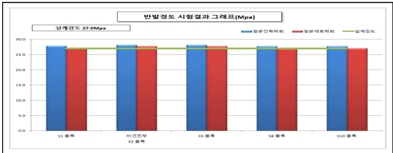
【그림 69.7】 반발경도시험 측정결과
